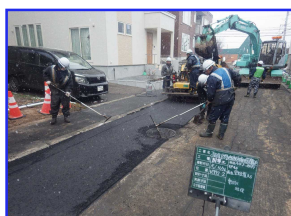
舗装敷均し
